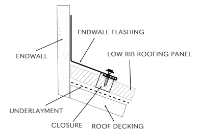
ENDWALL
