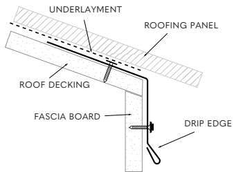
DRIP EDGE
